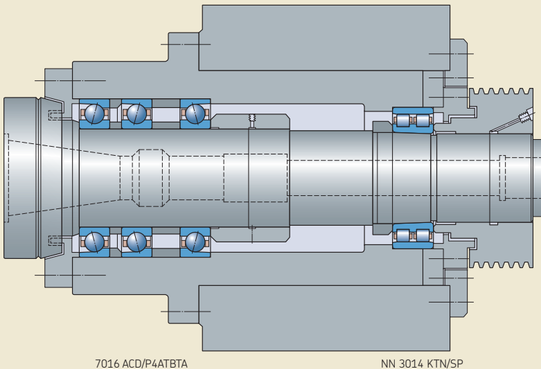
Riemengetriebene CNC-Drehspindel
